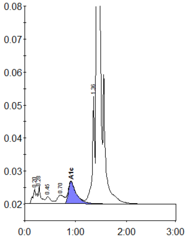
Peak table - ID: 10591722
